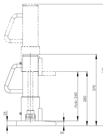
JHS 10 | Art.No. 01 020 101-O | Seitenansicht | Side view
