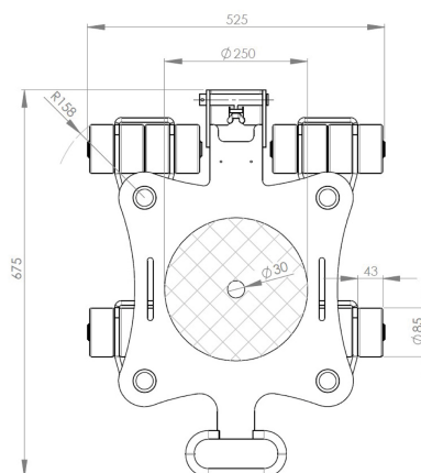
JKB 6 K | Art.No. 14 061 085-PJ Draufsicht | Top view
