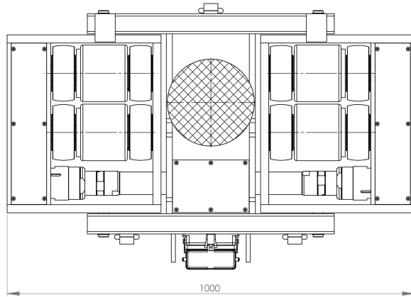
JLA-p 15/30 G | Art.No. 22 150 140-V | Draufsicht | Top view
