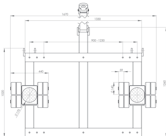
JTL 20 G | Art.No. 12 202 140-V | Draufsicht | Top view
