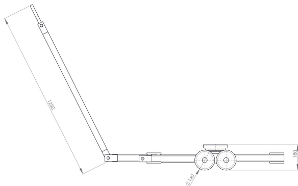
JTL 20 G | Art.No. 12 202 140-V | Seitenansicht | Side view
