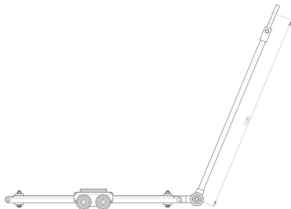
JTLB 14 K | Art.No. 12 121 085-D | Seitenansicht | Side view
