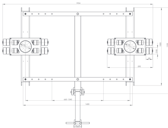
JTLB 14 K | Art.No. 12 121 085-D | Draufsicht | Top view
